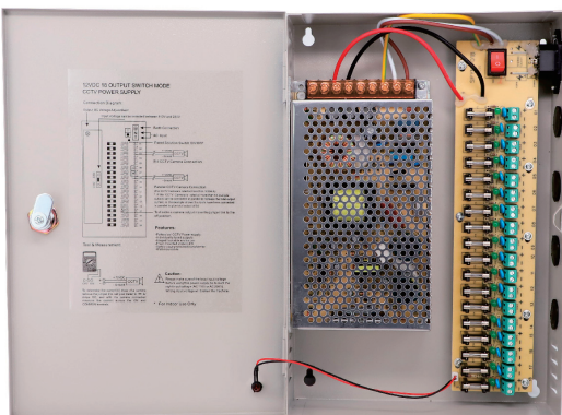
12V20A 18CH Power Box
